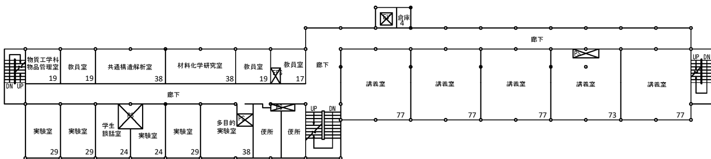
物質工学科・一般講義棟 3 階平面図
