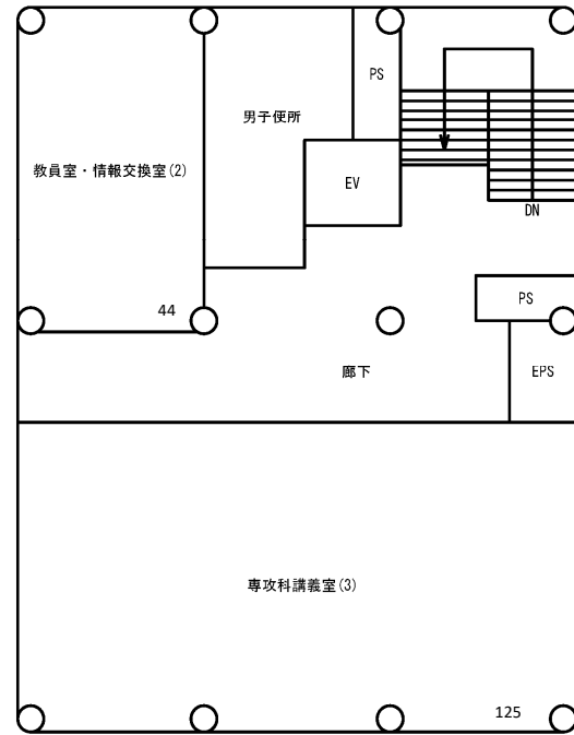
専攻科・総合教育棟4階平面図
