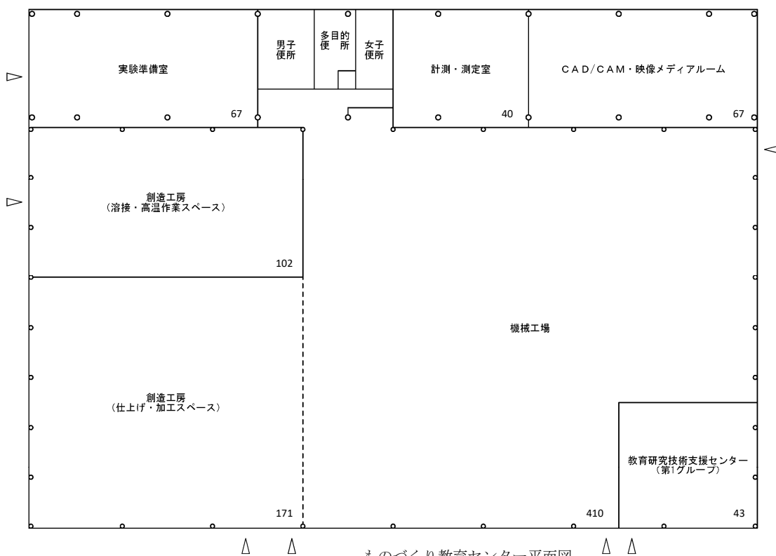
ものづくり教育センター平面図
