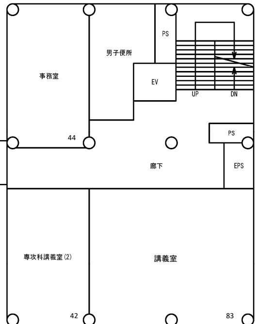
専攻科・総合教育棟3階平面図
