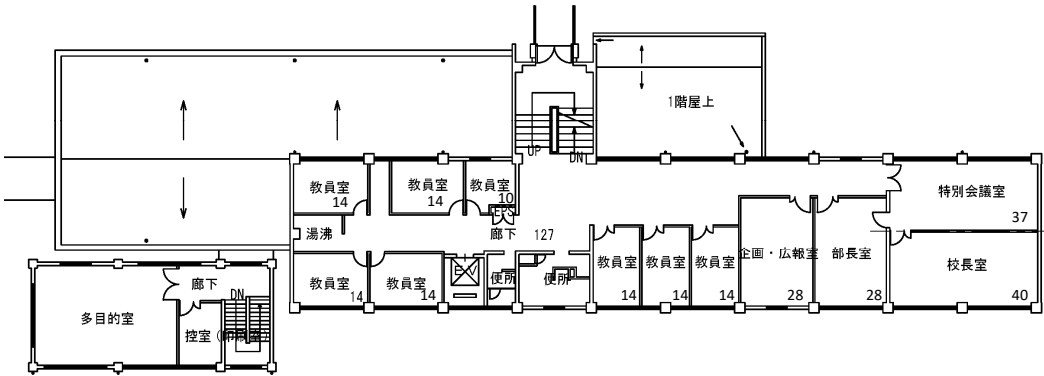
管理棟2階平面図
