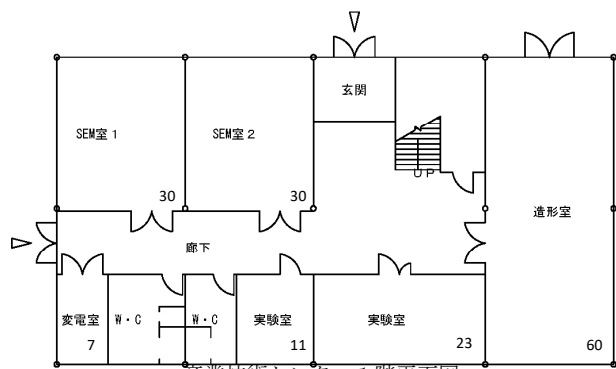
産業技術センター 1 階平面図
