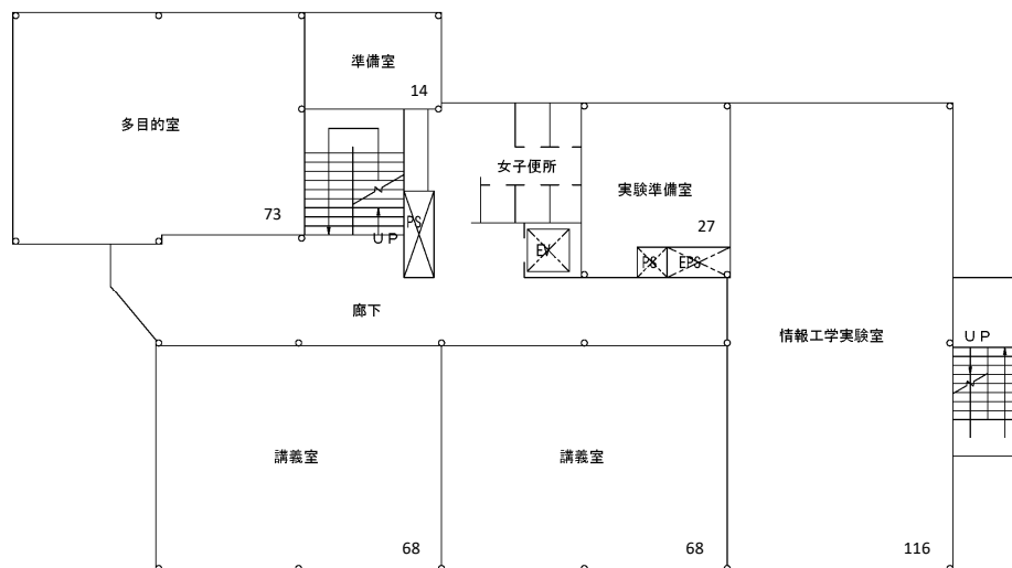
情報工学科棟2階平面図
