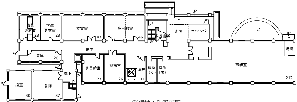
管理棟1階平面図
