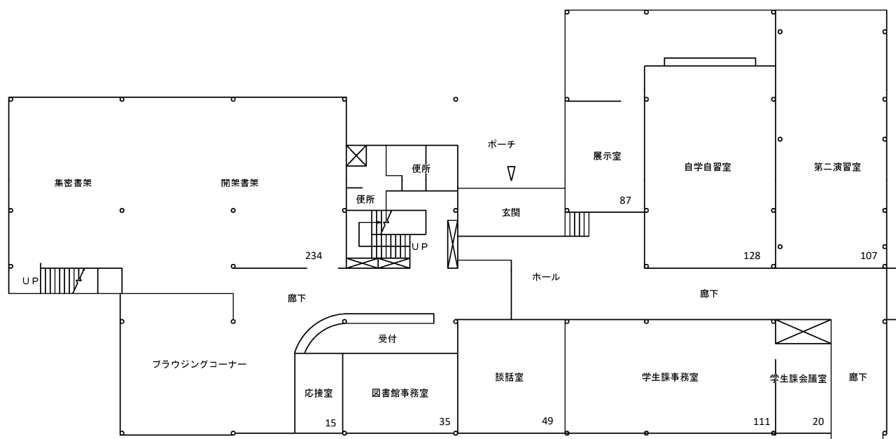
図書館 1 階平面図
