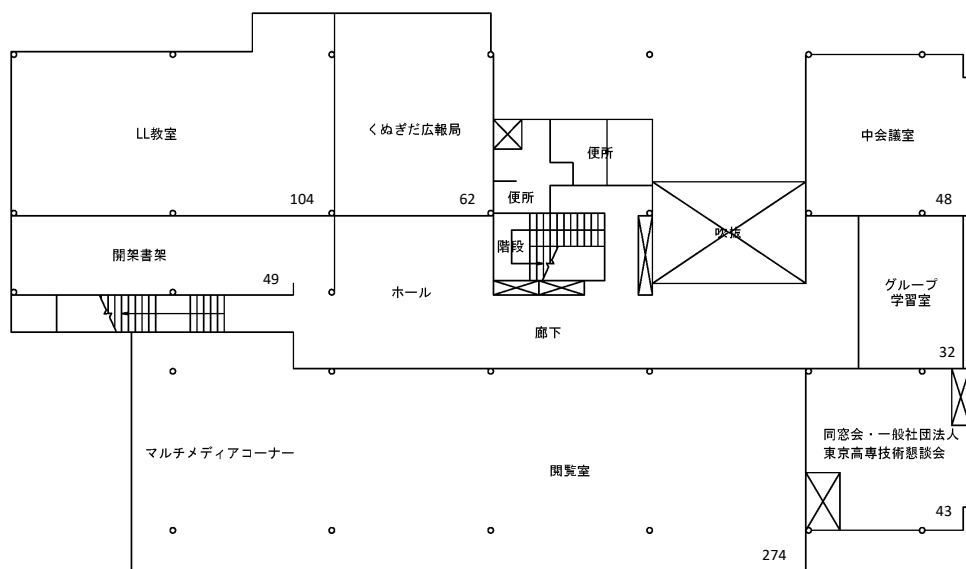
図書館 2 階平面図
